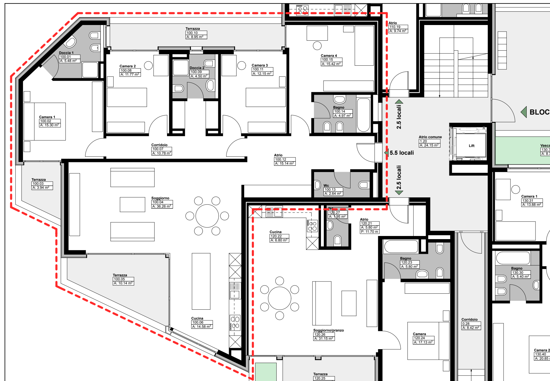
PIANTA APPARTAMENTO 1:100
